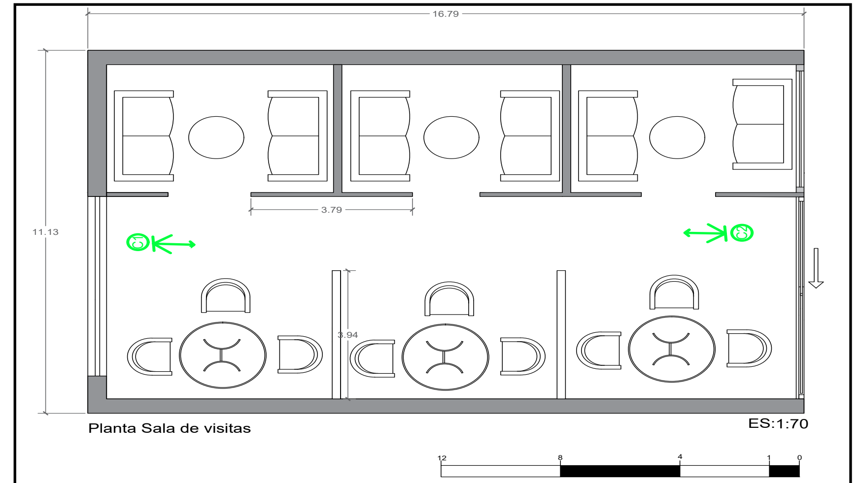
PLANTA SALA DE VISITAS
