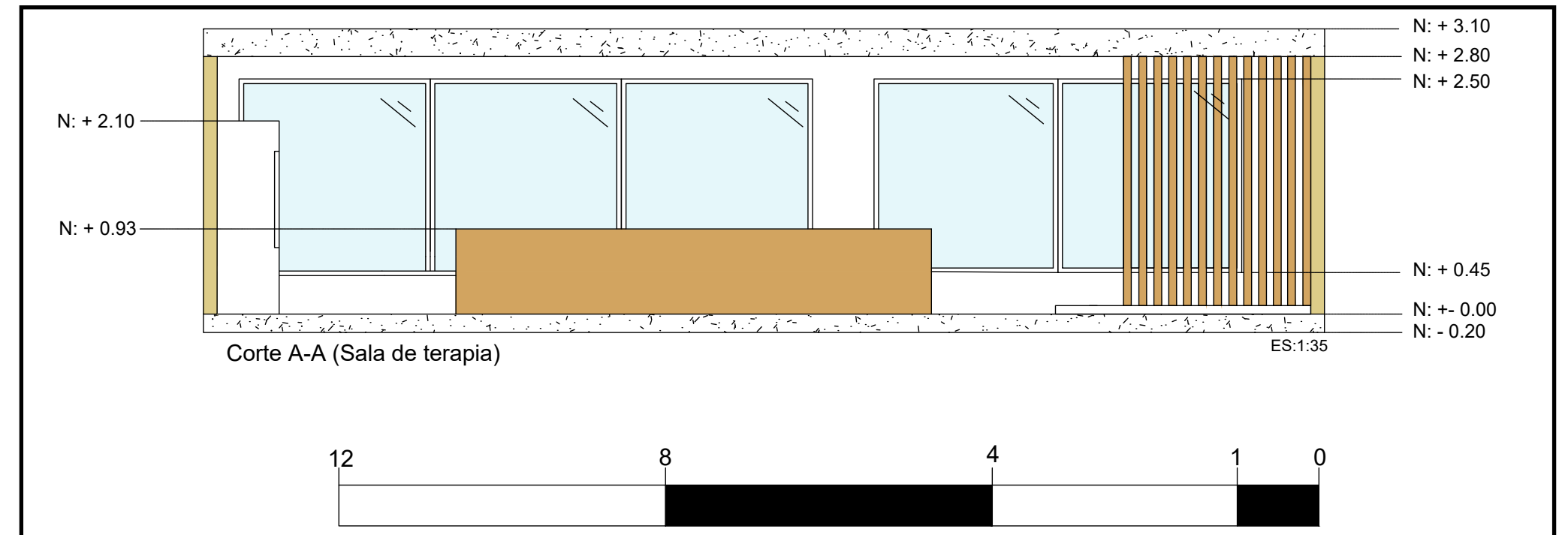
CORTE SALA DE TERAPIA
