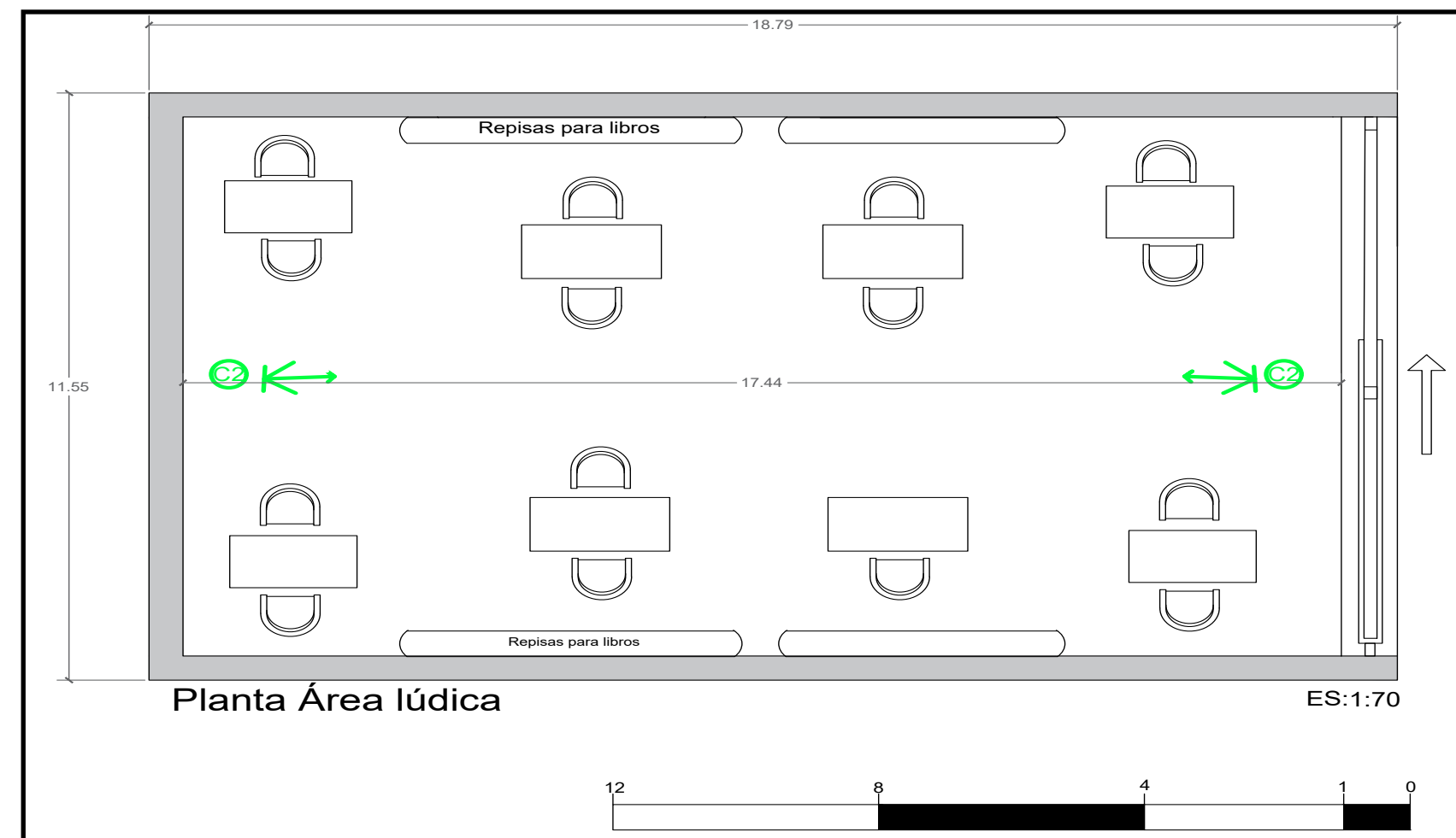
PLANTA ÁREA LÚDICA
