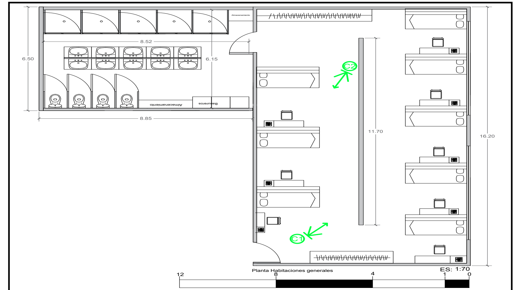
PLANTA HABITACIÓN GENERAL
