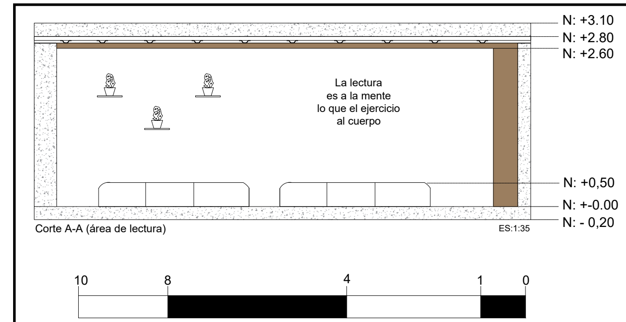
CORTE SALA DE LECTURA
