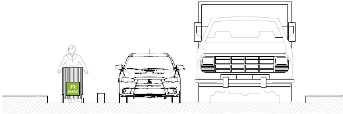
Figura 4.1: Detalle de la caminera Calle Roberto Crespo.
