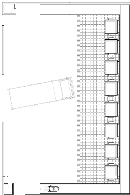
Figura 4.3: Vista en Planta Zona de Almacenamiento.
