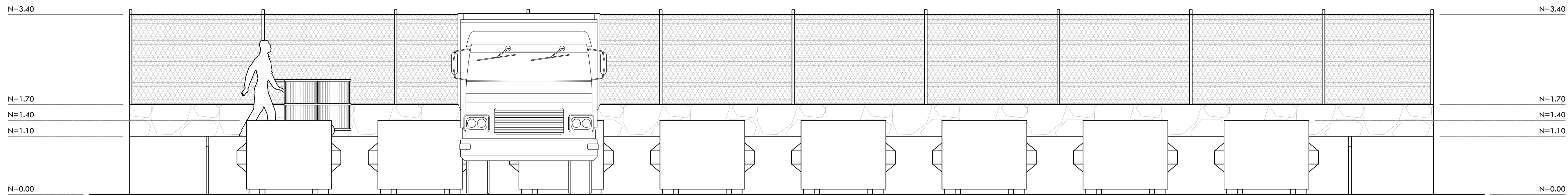
7 CORTE Y-Y' ESCALA 1_50
