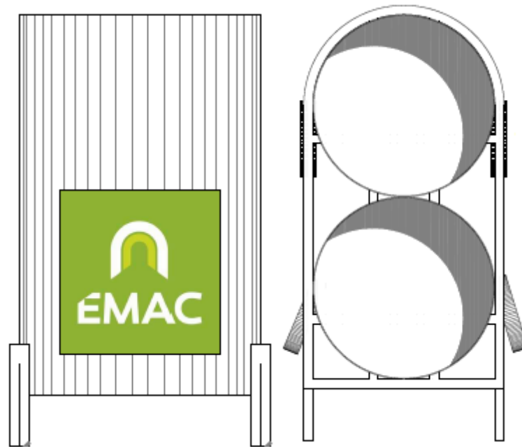
Figura 4.2: Detalle Carretilla Prototipo.
