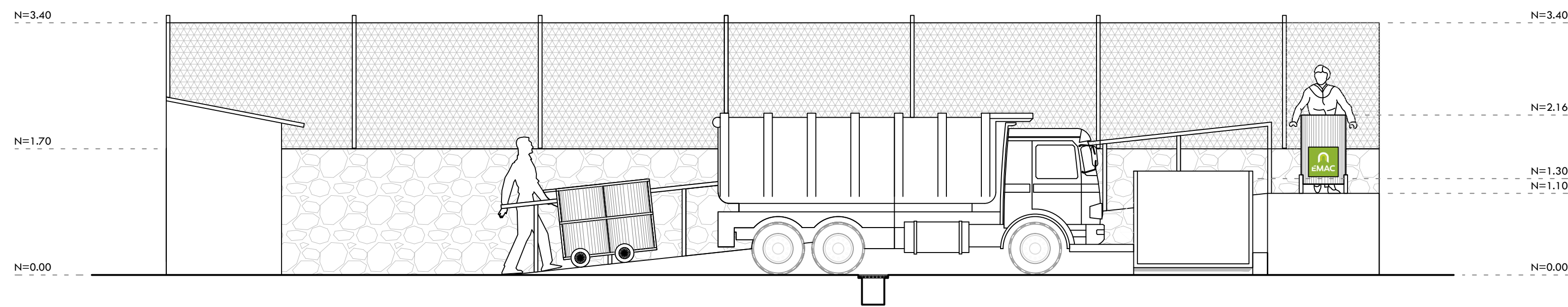
5 CORTE X-X' ESCALA 1_50
