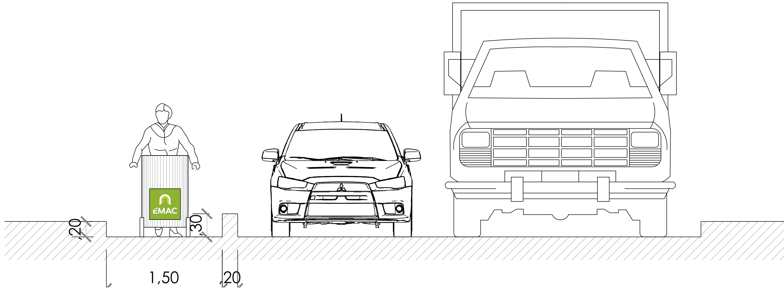
14 DETALLE DE CAMINERA CALLE ROBERTO CRESPO (CORTE) ESCALA 1_25
