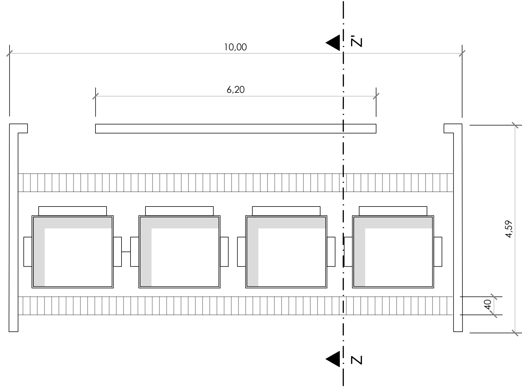
11 ZONA DE ALMACENAMIENTO INTERMEDIO (PLANTA) ESCALA 1_50
