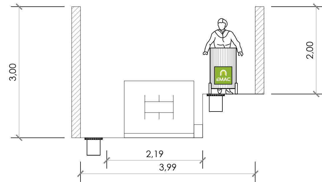
12 CORTE Z - Z' ESCALA 1_50
