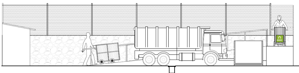
Figura 4.4: Vista en Corte Zona de Almacenamiento.
