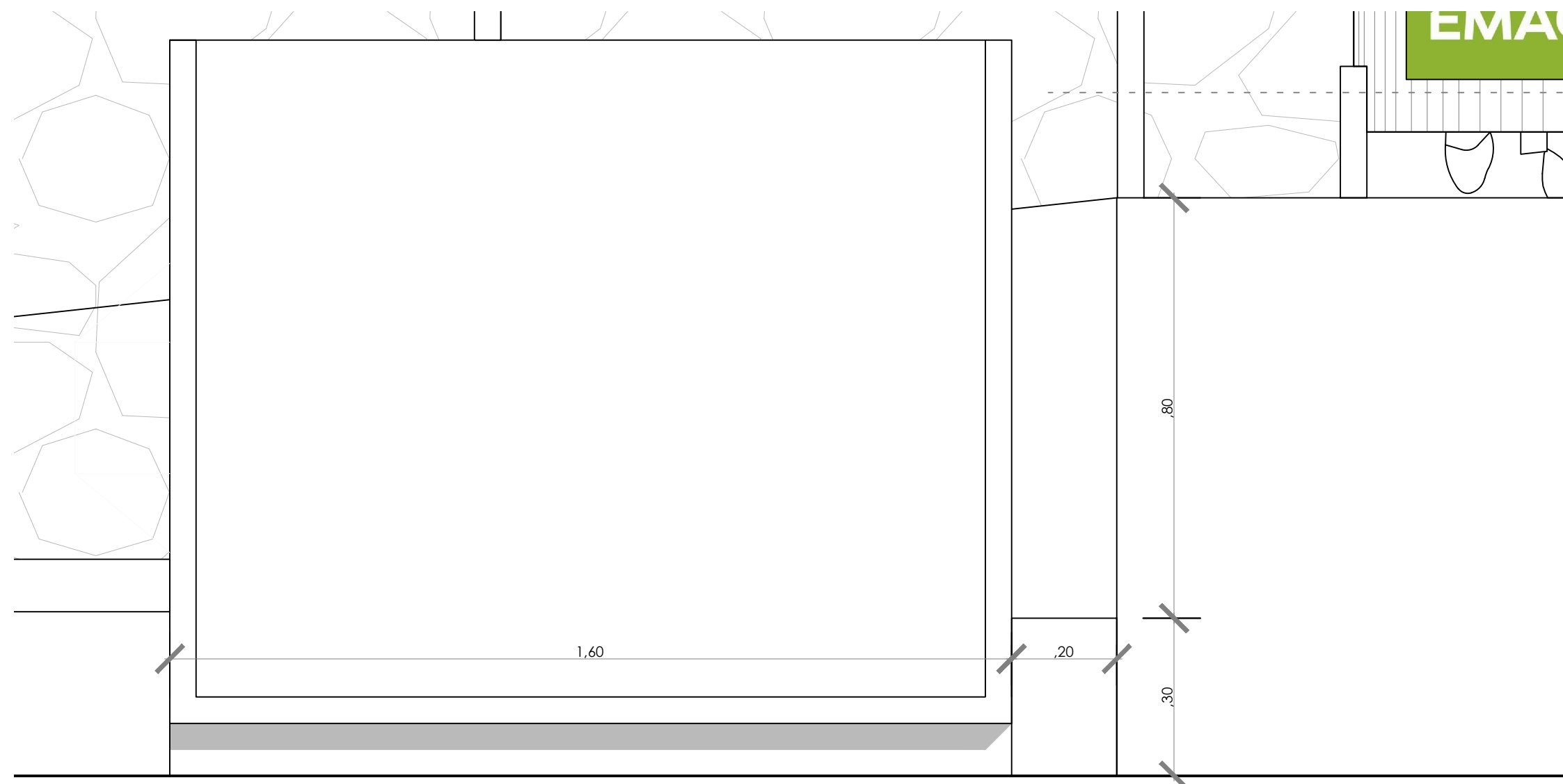
9 DETALLE DE BORDILLO DE HORMIGÓN PROTECTOR ESCALA 1_10
