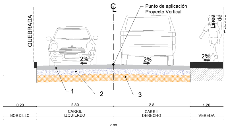
Figura 14: Sección transversal SECCION TRANSVERSAL
