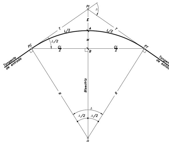
Figura 1: Elementos geométricos de la curva circular simple
