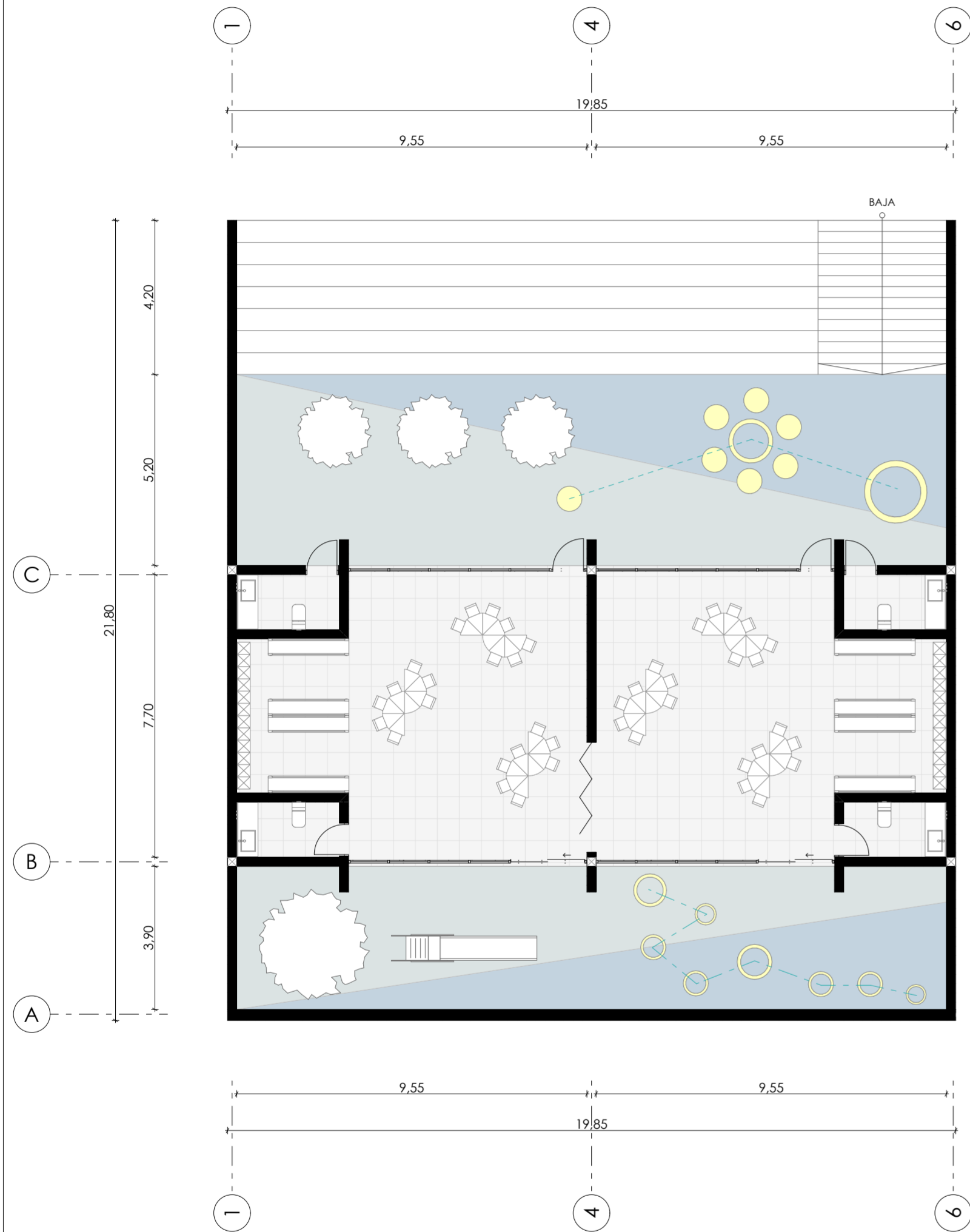
AMPLIACIÓN EDUCACIÓN INICIAL N - 3,40 ESC 1:125
