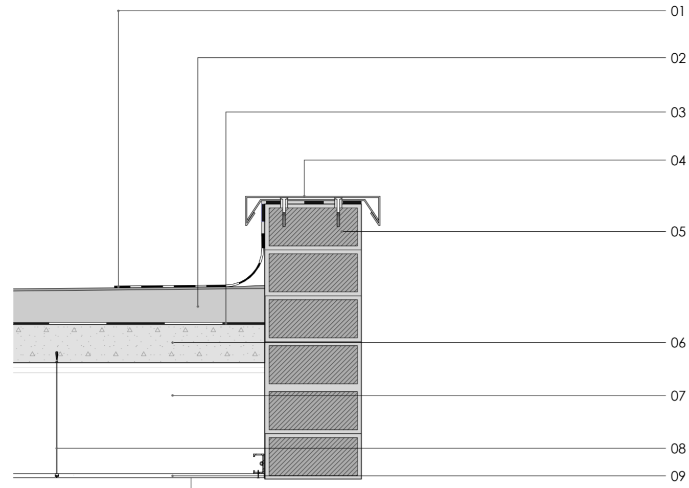
DETALLE 1 ESC 1:10
