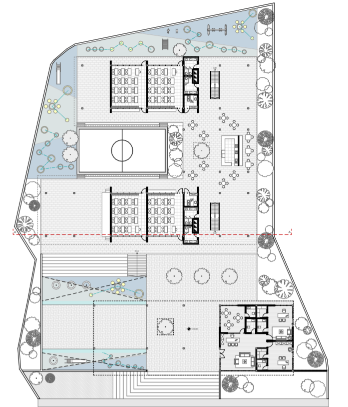
Planta Referencia Sección A-A
