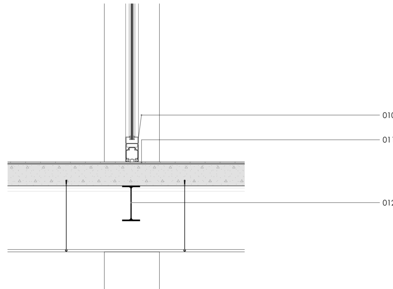
DETALLE 2 ESC 1:10
