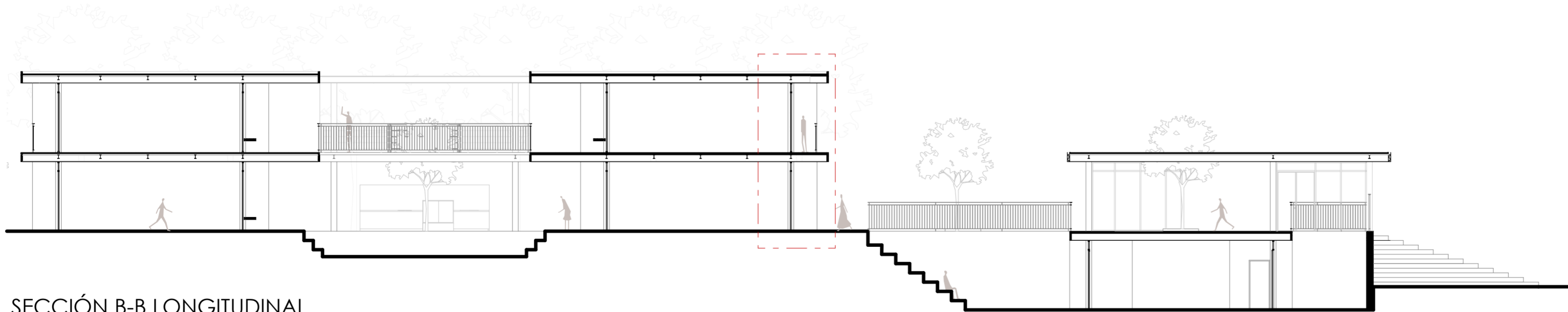
SECCIÓN A-A TRANSVERSAL BLOQUE EDUCACIÓN BÁSICA ESC 1:100
