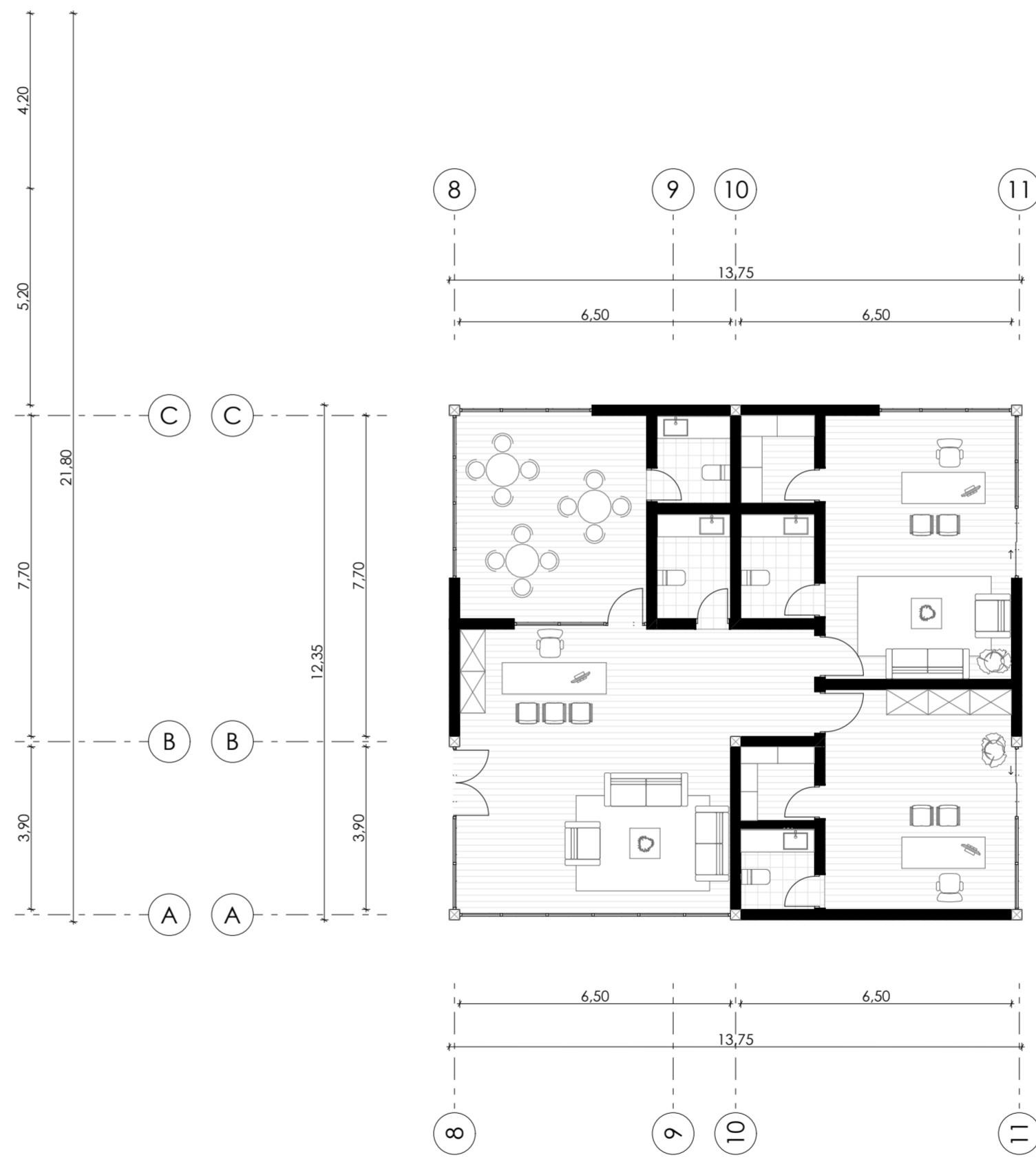
AMPLIACIÓN ADMINISTRACIÓN N + 0,00 ESC 1:125
