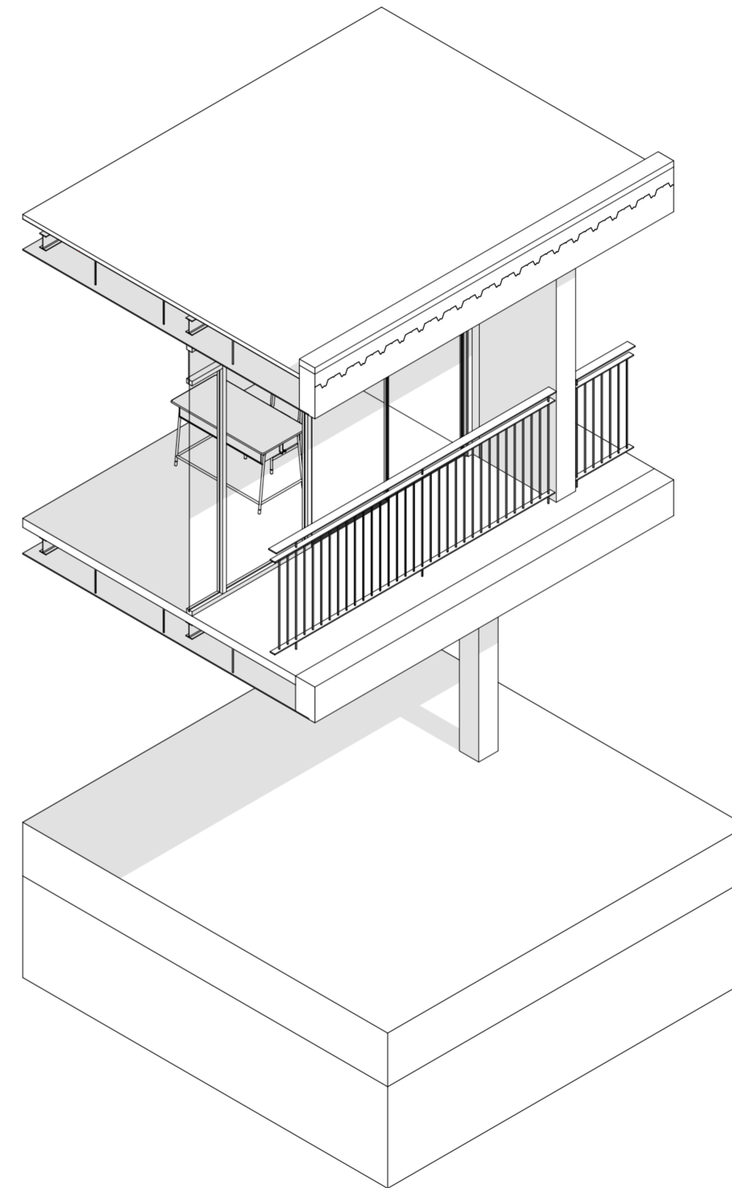
SECCIÓN AXONOMÉTRICA
