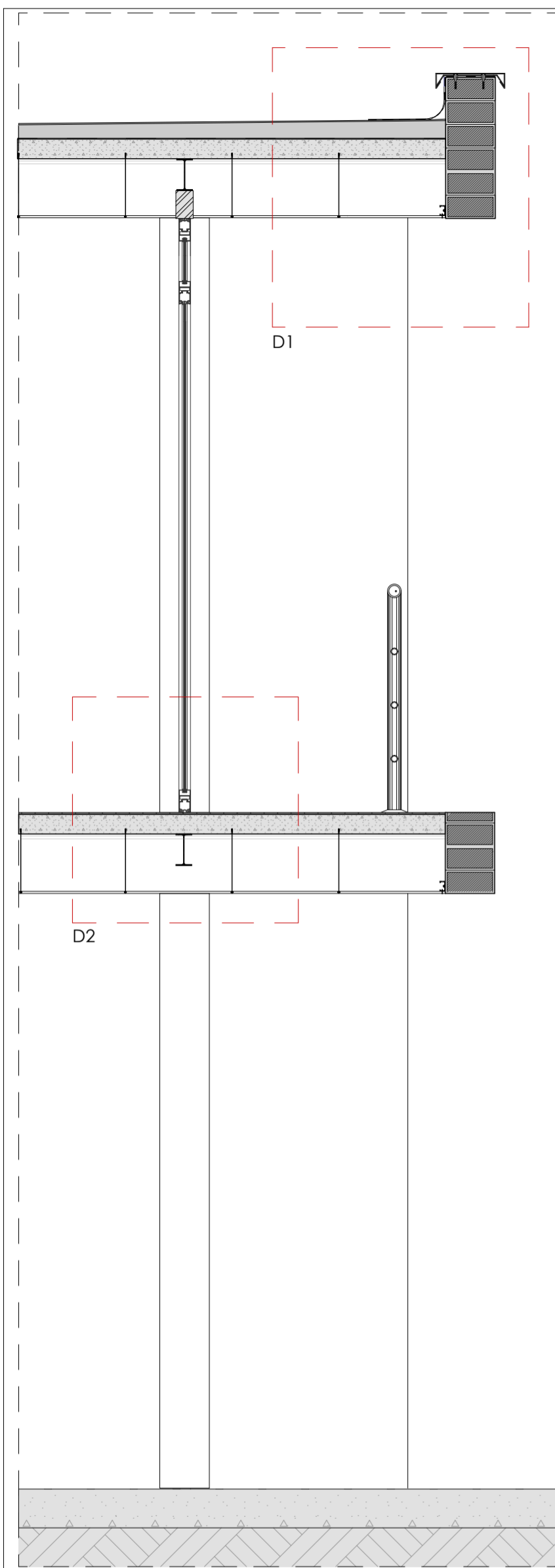
SECCIÓN CONSTRUCTIVA ESC 1:25
