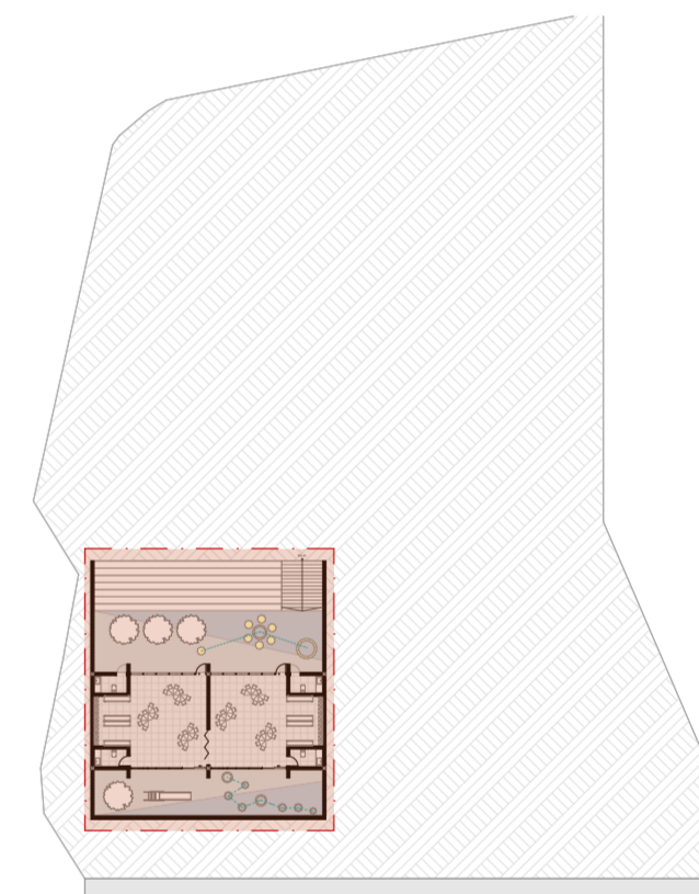
Planta Referencia Ampliación Educación Inicial
